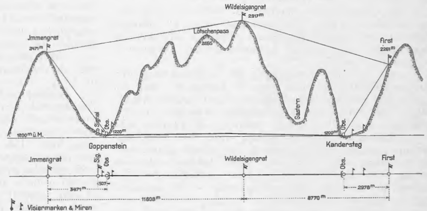
Abb. 2. Längensprofil der oberirdischen Absteckung. — Längen 1 : 200 000, Höhen 1 : 50 000.
